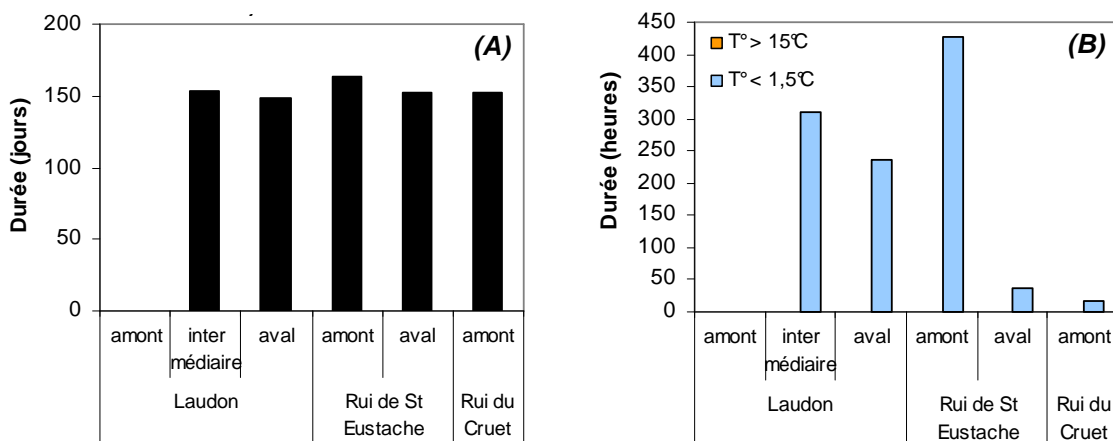
Figure 24 : Durée totale en jours de la phase embryo-larvaire de la vie sous graviers (de la fécondation à l'émergence) (A) et durée en heures des séquences maximales durant laquelle la température est restée en dessous de 1,5°C et au dessus de 15°C pendant la période de développement embryo-larvaire (B) sur les stations concernées par le suivi thermique annuel : 3 sur le Laudon et les 3 sur ses affluents.
